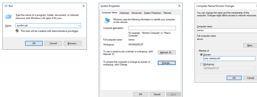
Obr. 3.1: Pridanie počítača do domény
